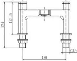
Bath Filler NV218 NV218-MB NV218-BB
