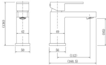
Basin Mixer NV216 NV219-MB NV216-BB
