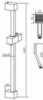
Mayfair Slide Rail Kit NV194 NV194-MB NV194-BB
