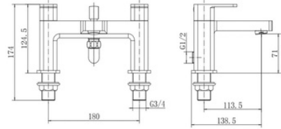
Bath Shower Mixer NV220 NV220-MB NV220-BB
